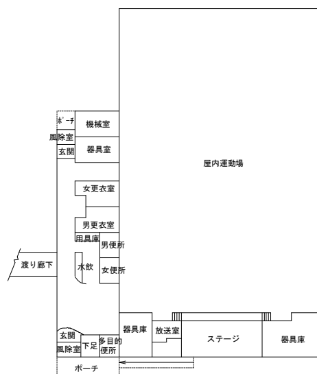
平面図
