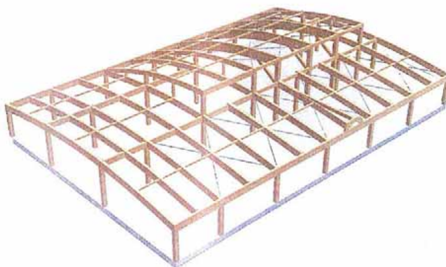
木造で筋違いのないラーメン構造
